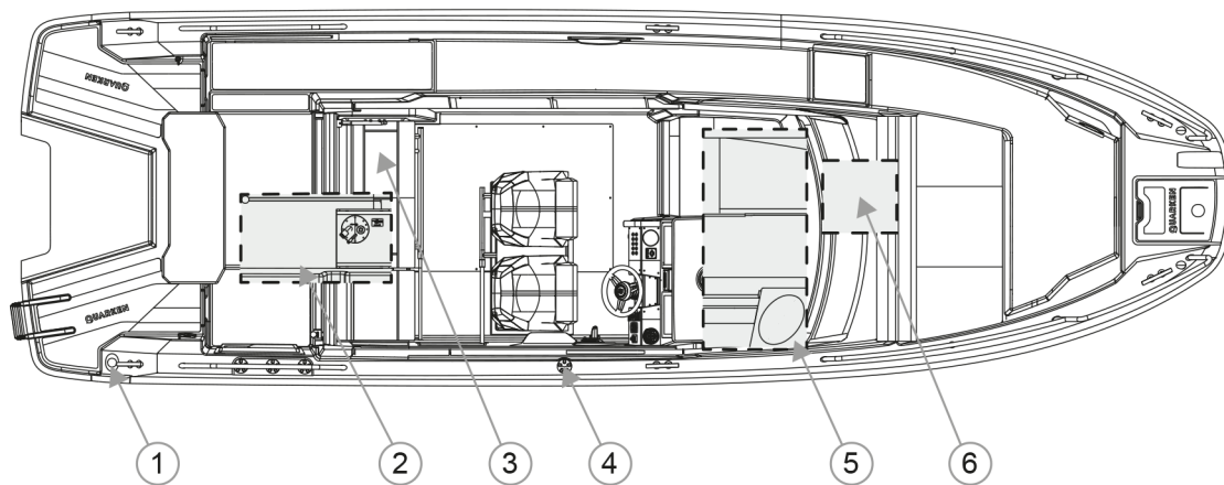
Abbildung 4.16 Frischwassersystem
