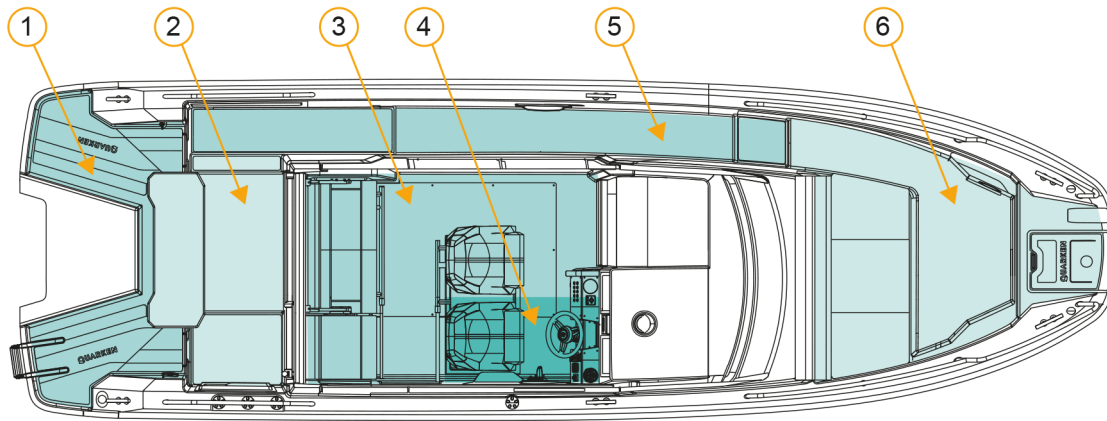
Abbildung 3.1 Deckbereiche
