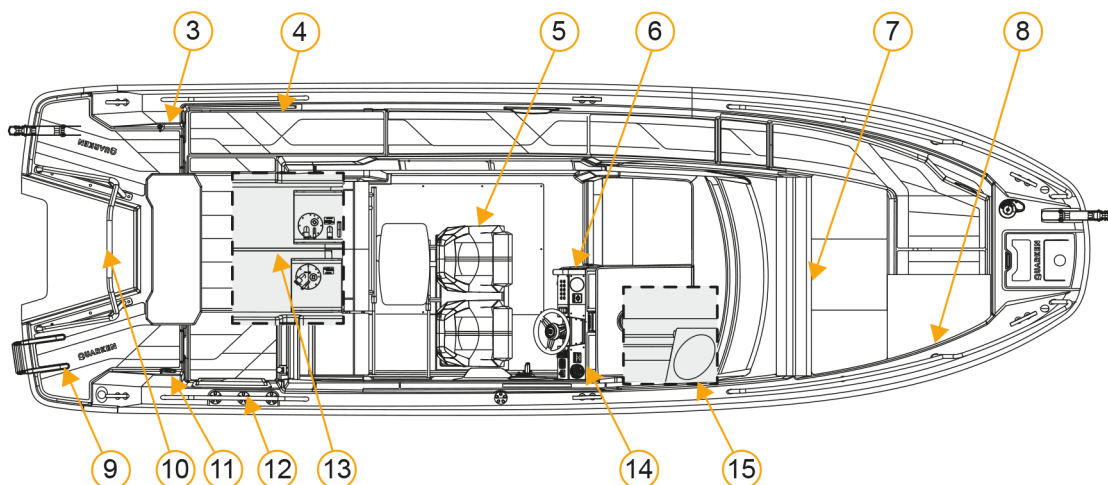
Abbildung 2.4 Sicherheitshinweise an Bord
