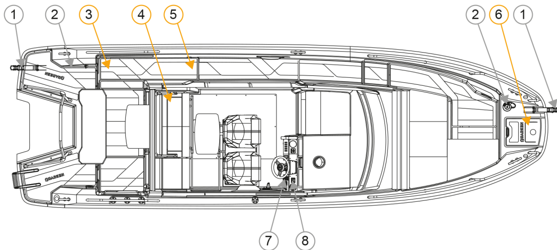
Abbildung 4.11 Ankerwinde
