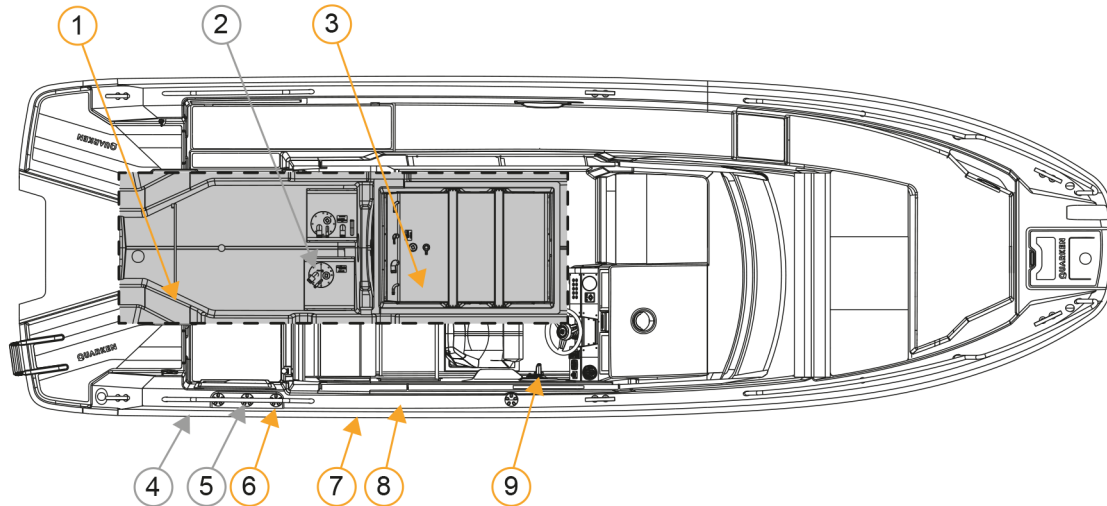
Abbildung 4.1 Kraftstoffsystem
