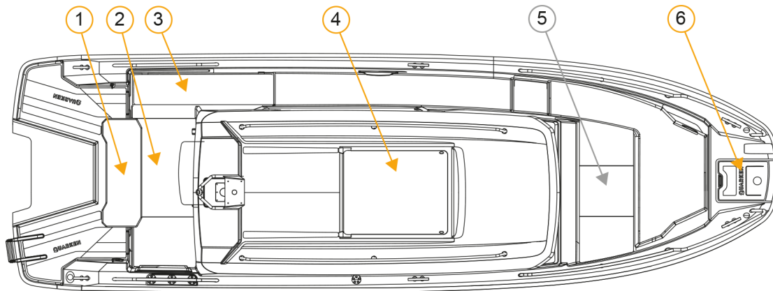
Abbildung 4.13 Fenster, Türen und Luken
