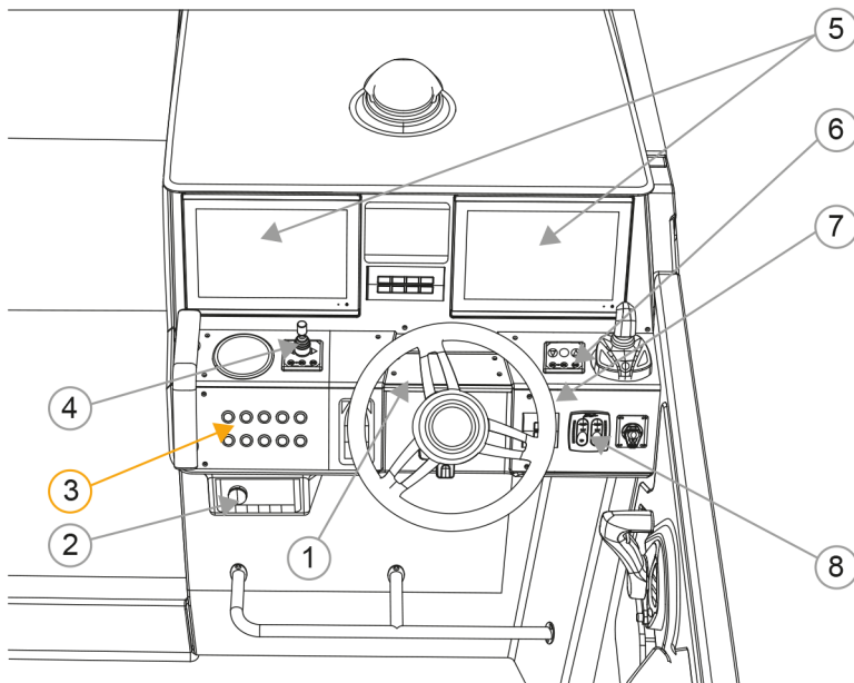
Abbildung 4.5 Bedienelemente der Steuerkonsole
