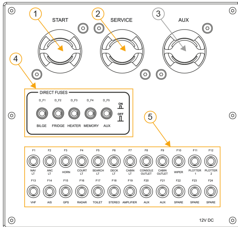
Abbildung 4.3 Hauptschalttafel
