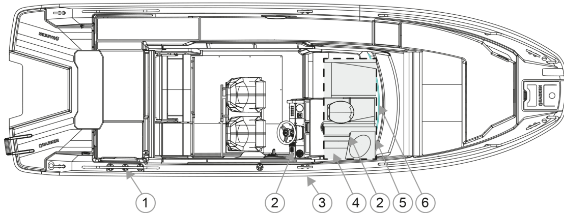
Abbildung 4.18 Komponenten des Heizgeräts
