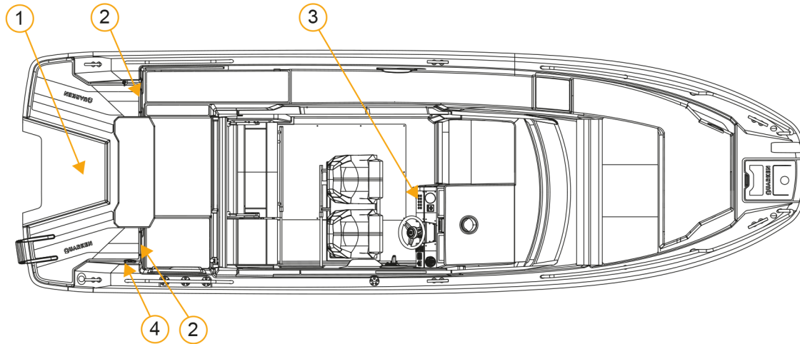
Abbildung 4.14 Abflusssystem
