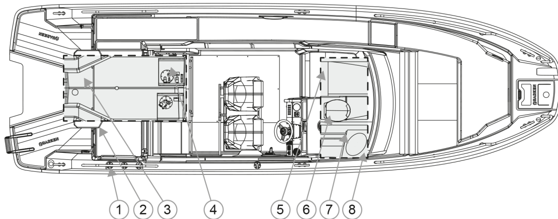
Abbildung 4.17 Komponenten des Abwassersystems
