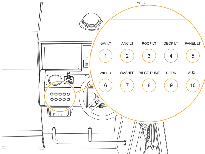
Abbildung 4.6 Bedienelemente auf dem Multifunktionspanel
