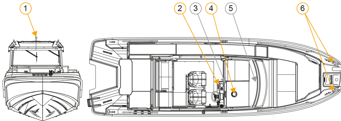
Abbildung 4.8 Komponenten des Navigationssystems
