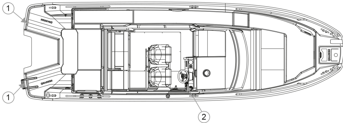
Abbildung 4.10 Trimmklappen
